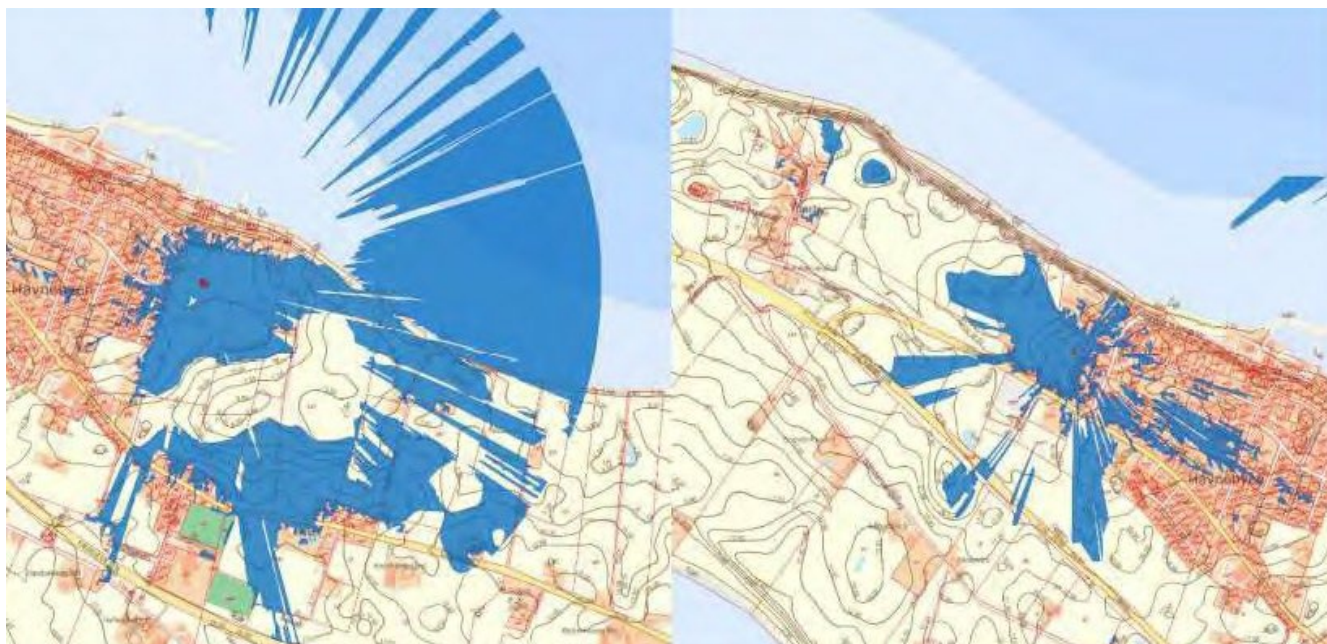
Synlighedsberegning af 8,5 meter høj bygning indenfor 1000 meter. Eksisterende rammelagt areal 1R2 til venstre og nyt rammelagt areal 1R6 til højre.
